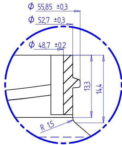
DETALLE A 2:1
